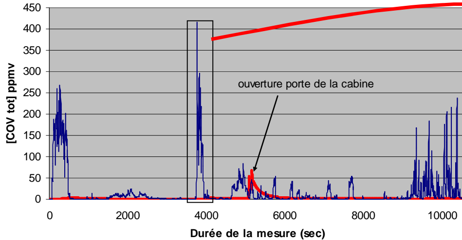
Mesure des COV tot pendant une opération DISCONTINUE de brassage de fosse
